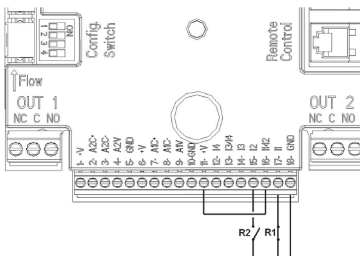
Схема 4: Пример подсоединения цифровых вводов
